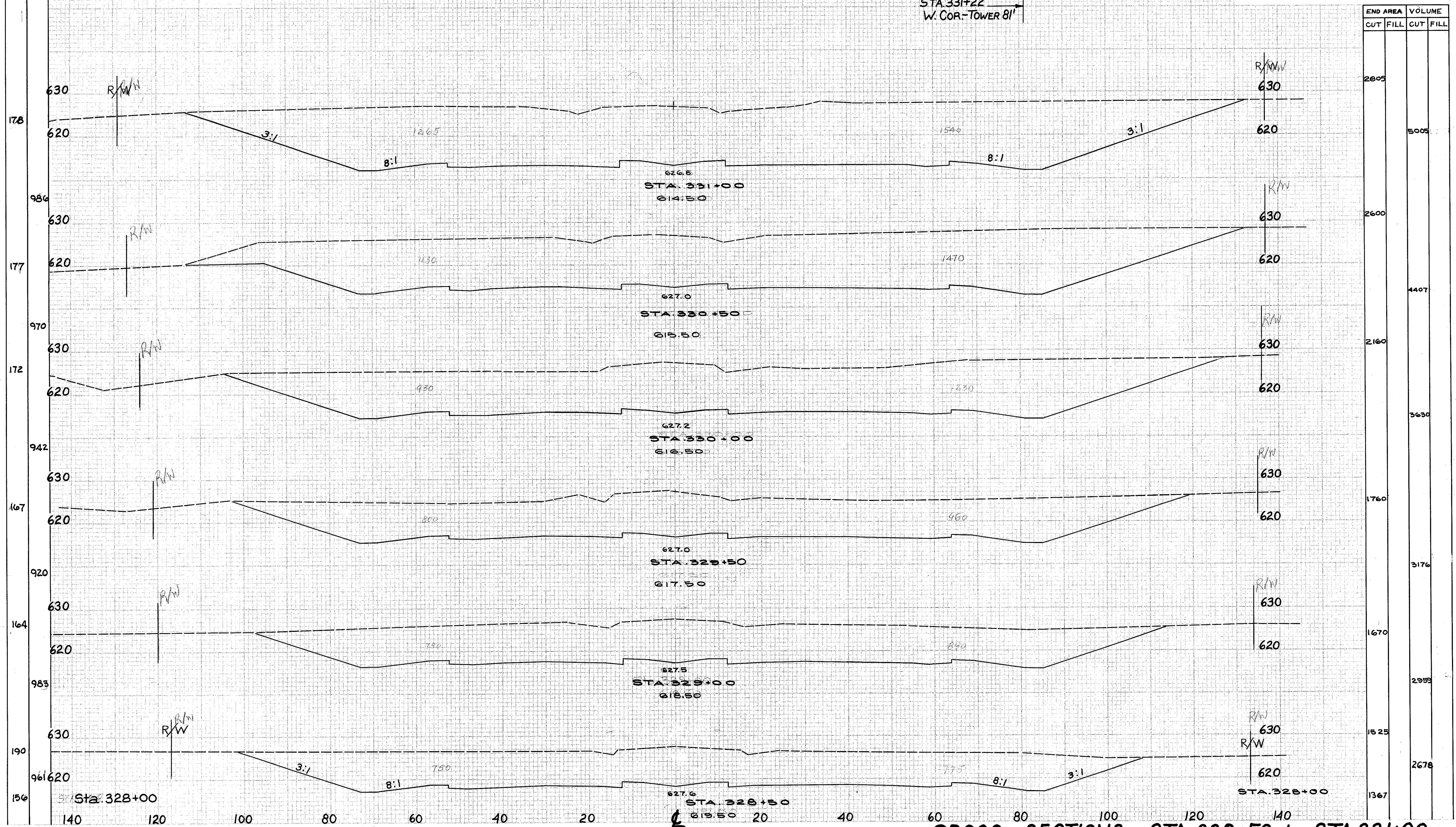
CROSS SECTIONS STA. 328+50 to STA. 331+00
