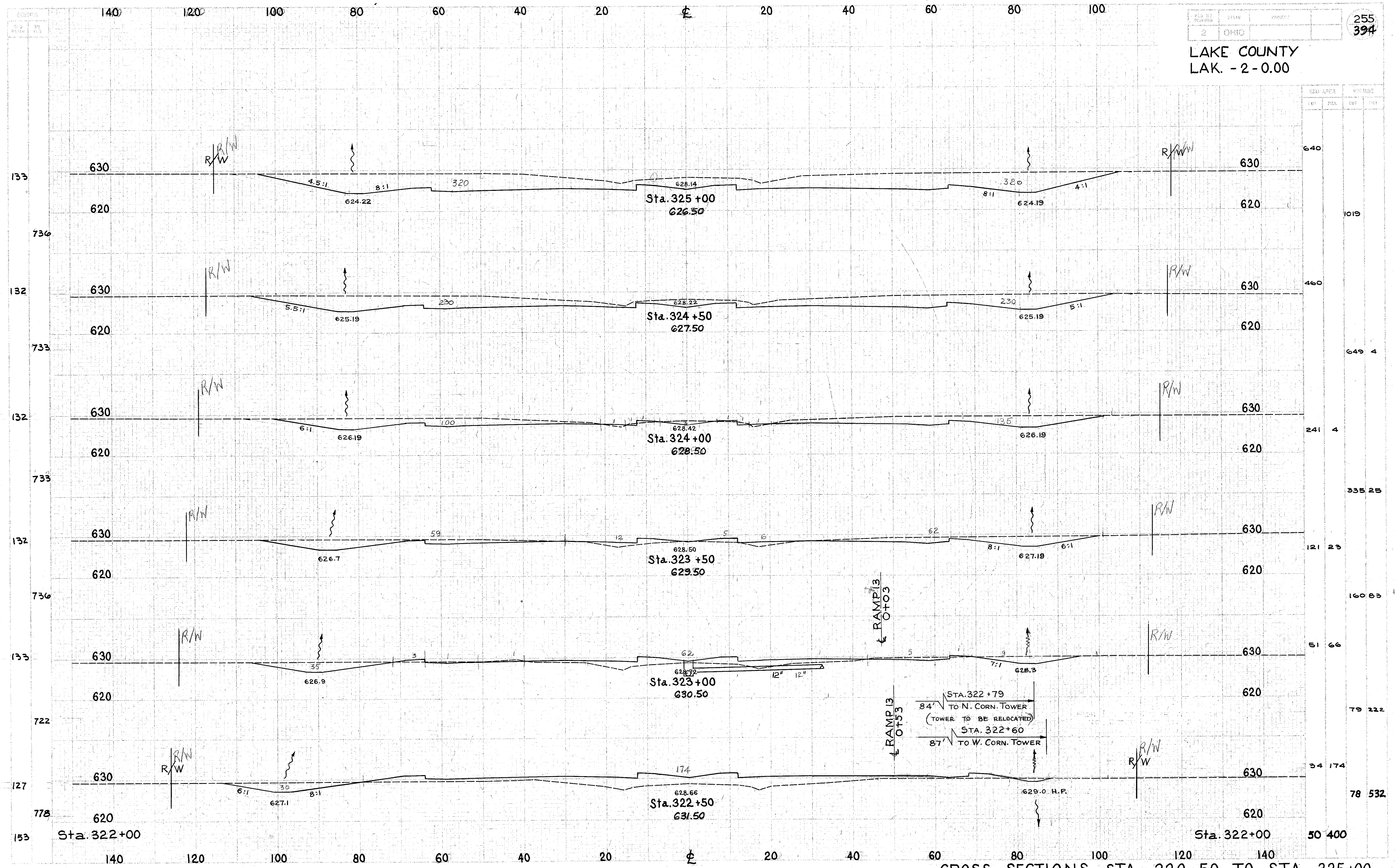
CROSS SECTIONS STA. 322+50 TO STA. 325+00
