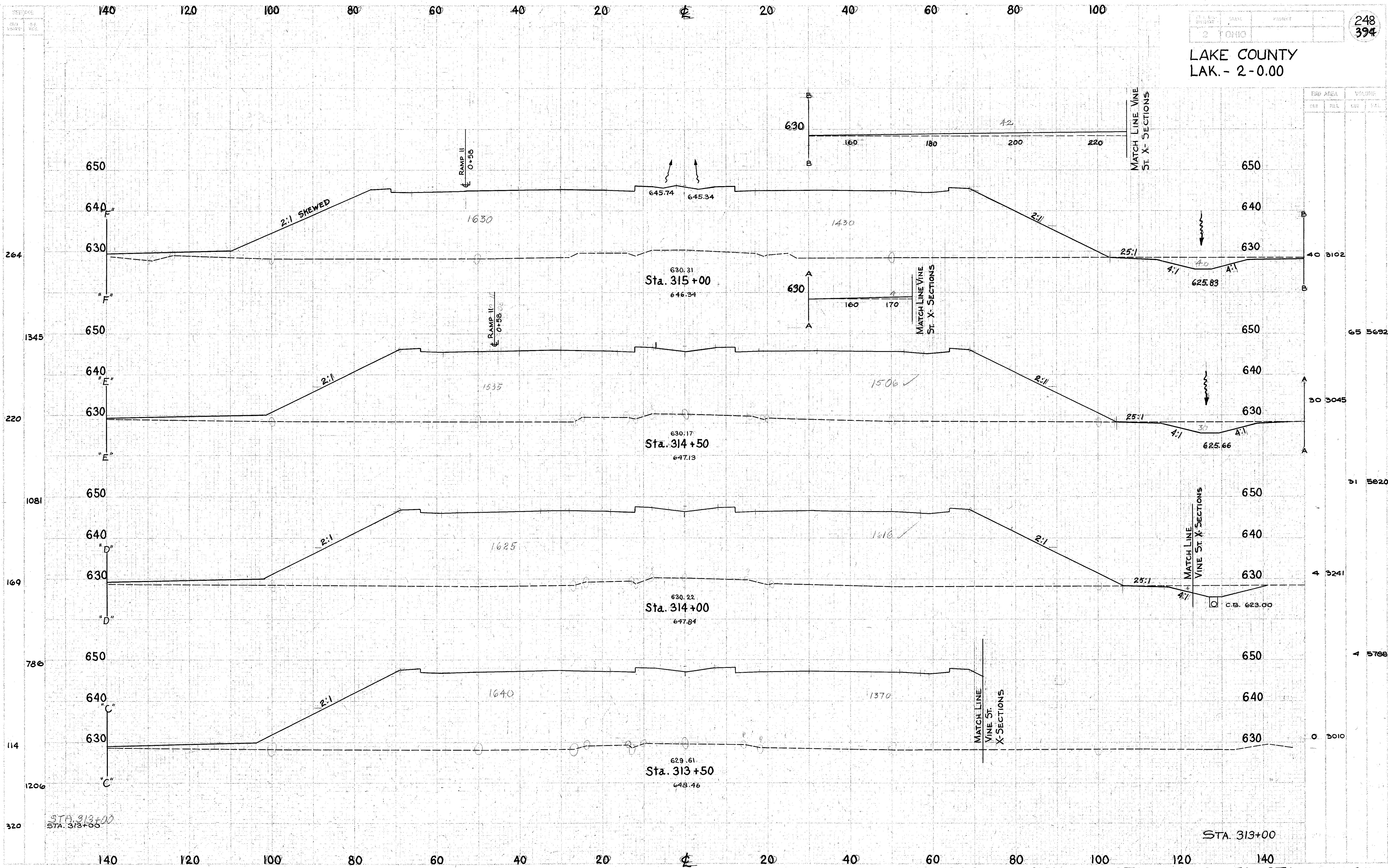
CROSS SECTIONS STA. 313+50 TO STA. 315+00
