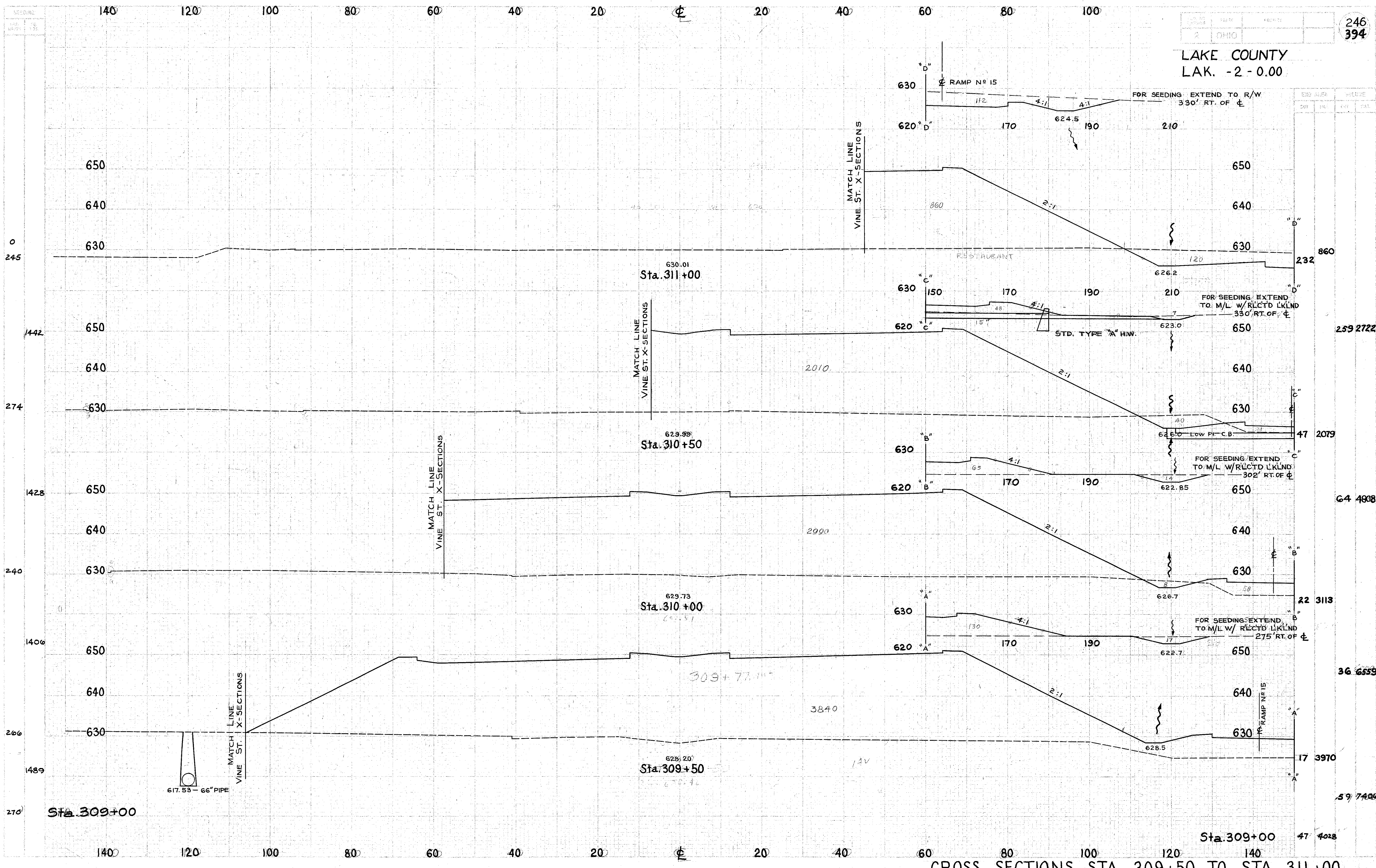
CROSS SECTIONS STA. 309+50 TO STA. 311+00
