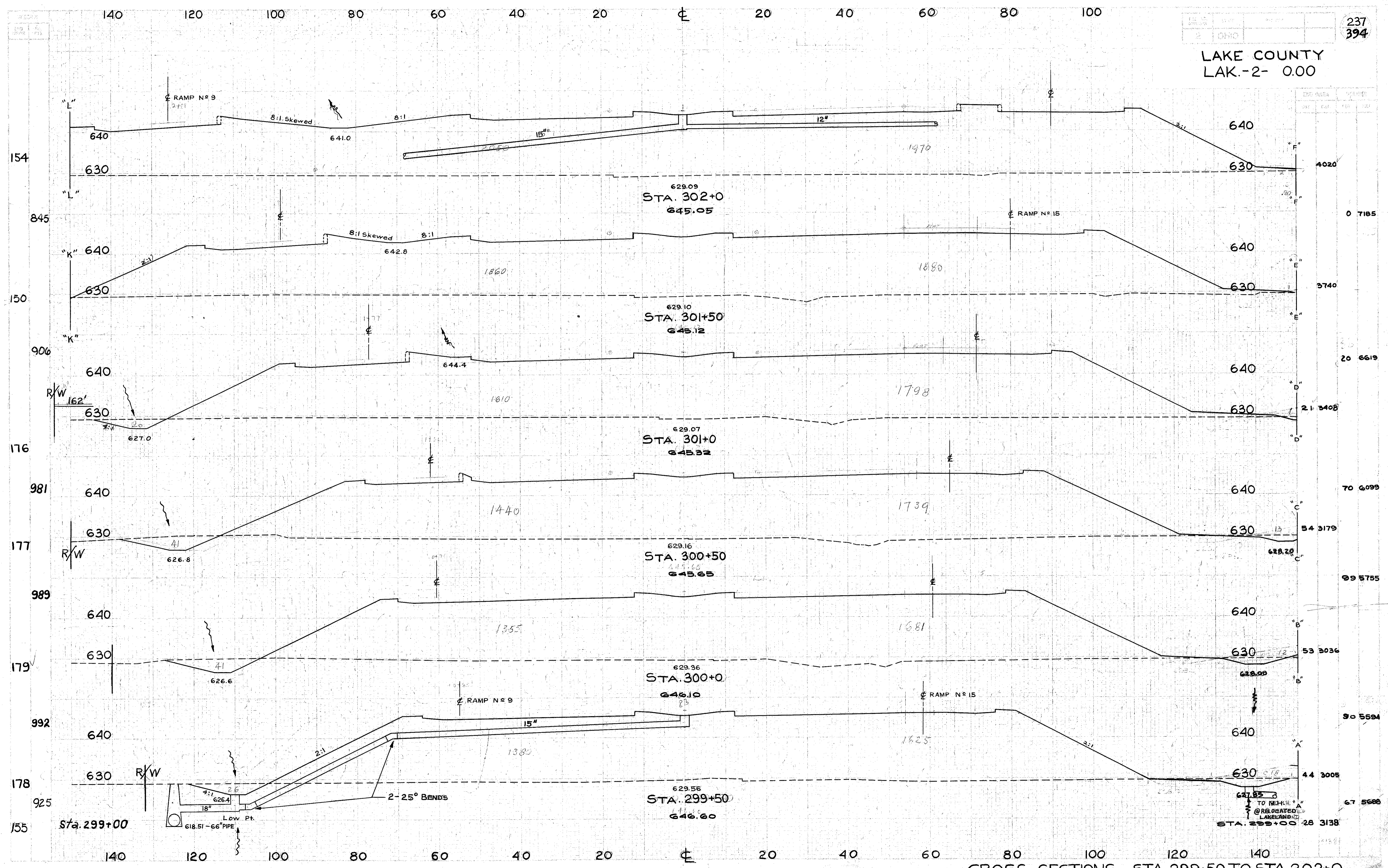
CROSS SECTIONS STA. 299+50 TO STA. 302+0
