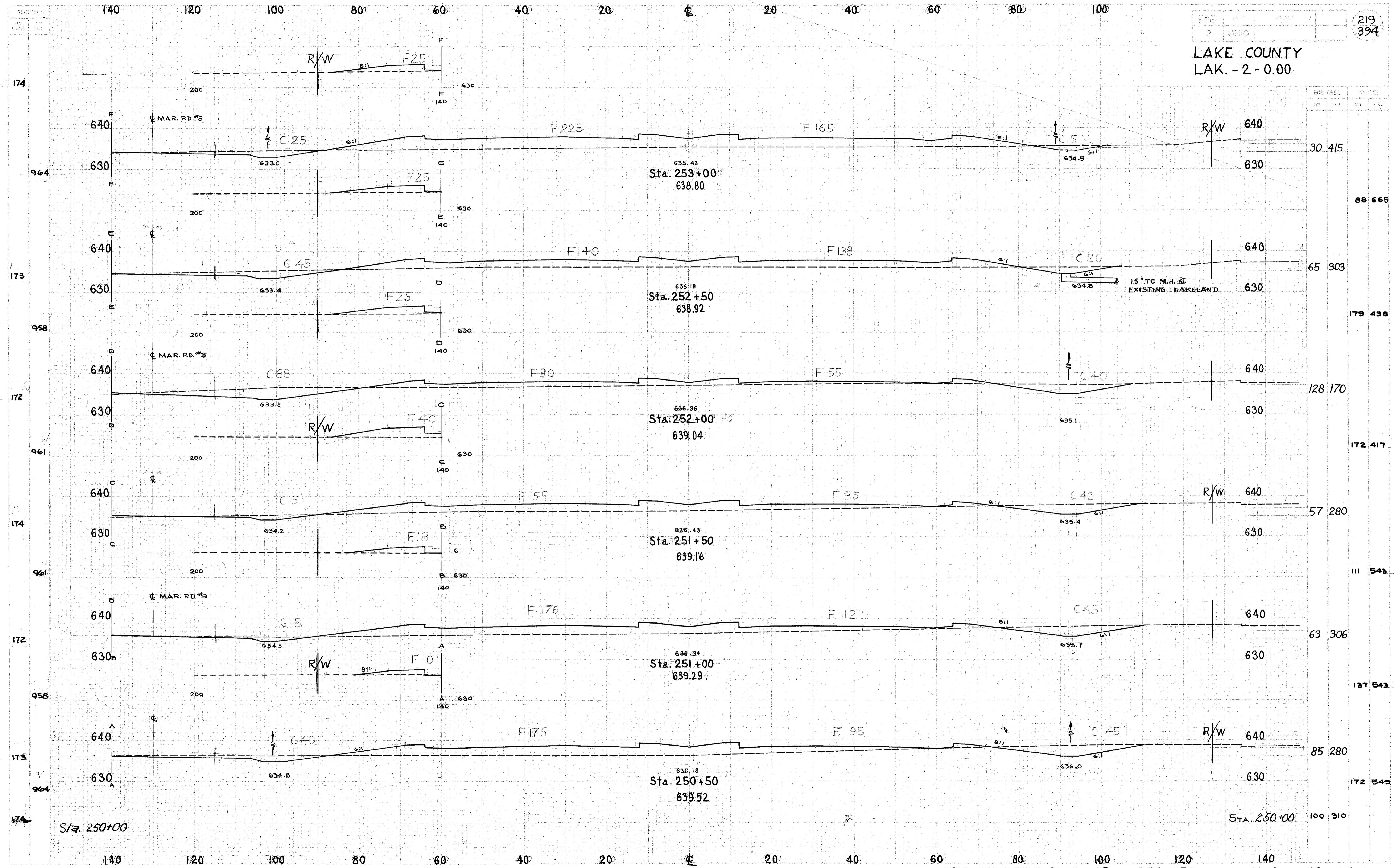
CROSS SECTIONS STA. 250+50 TO STA. 253+00
