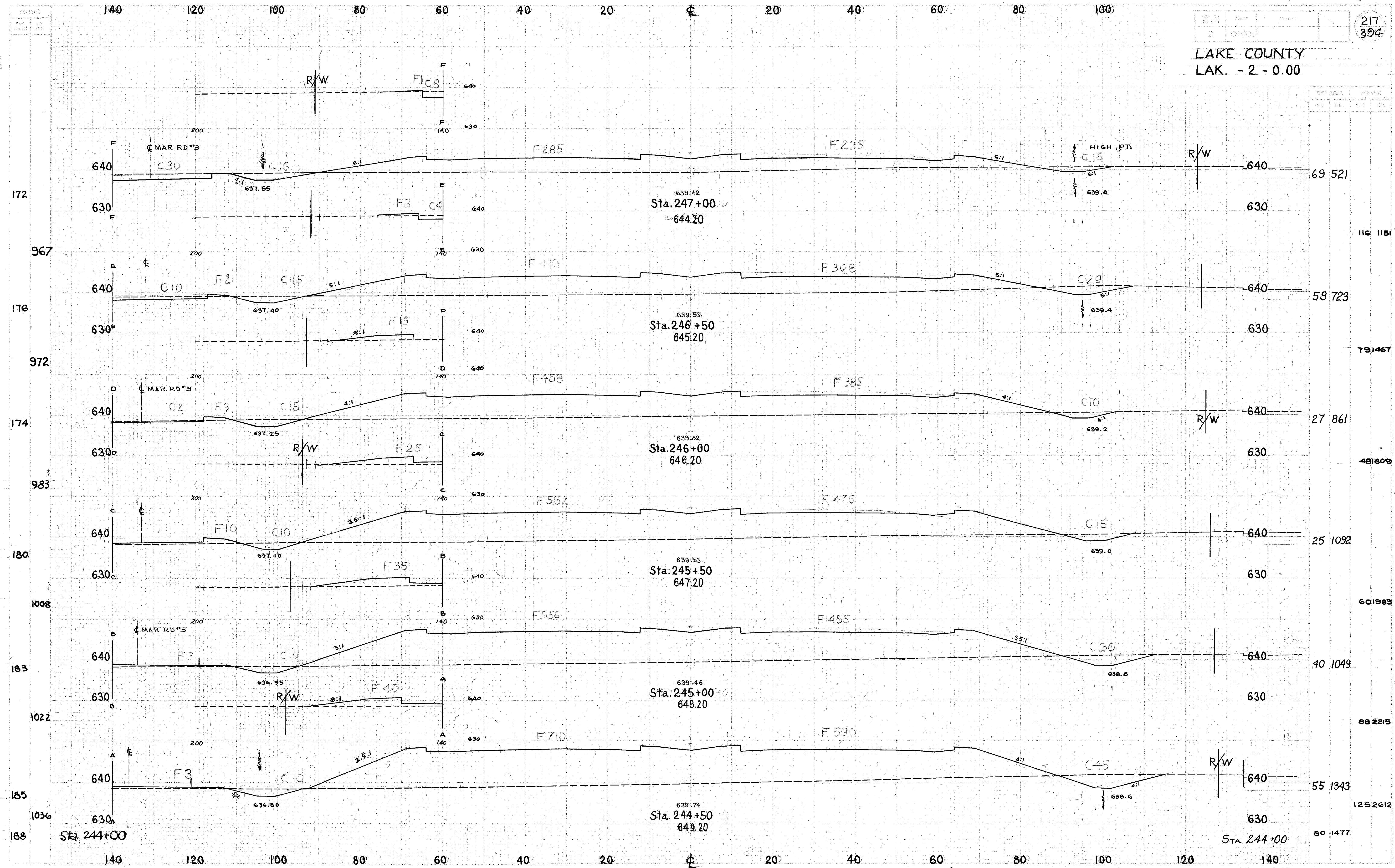
CROSS SECTIONS STA. 244+50 TO STA. 247+00
