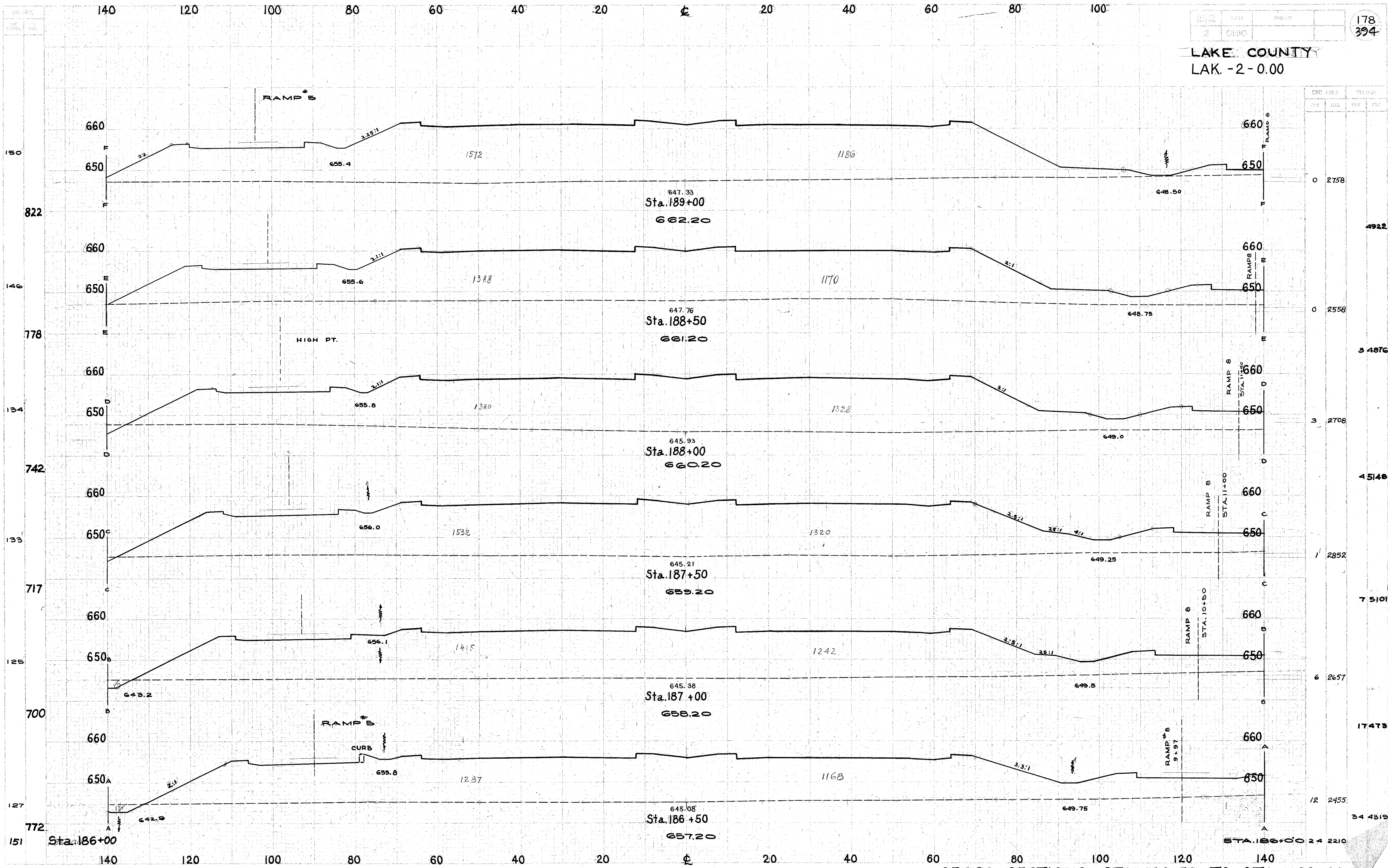
CROSS SECTIONS STA. 186+50 TO STA. 189+00
