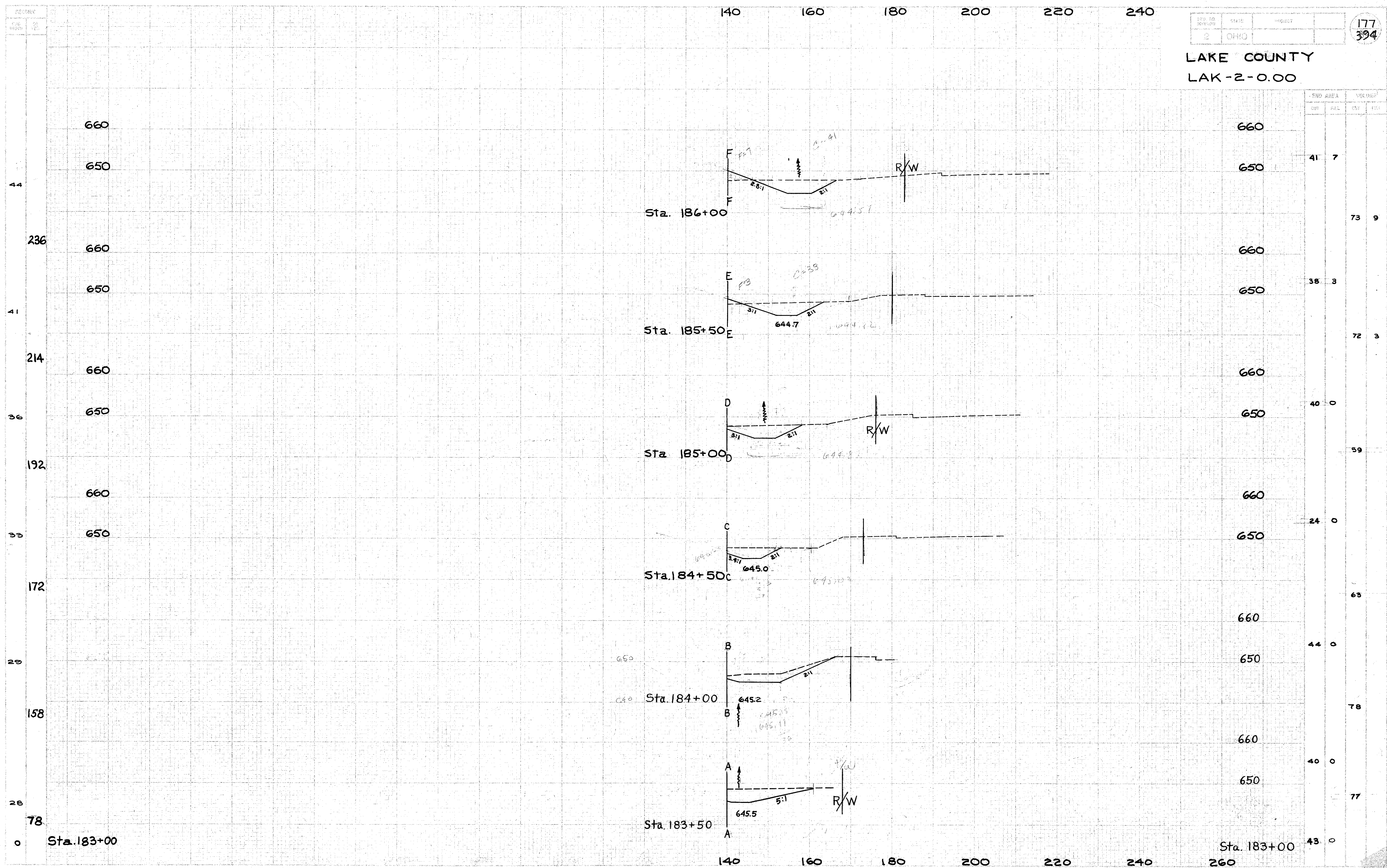
CROSS SECTION EXTENSIONS STA. 183+50 TO STA. 186+00 (RIG)
