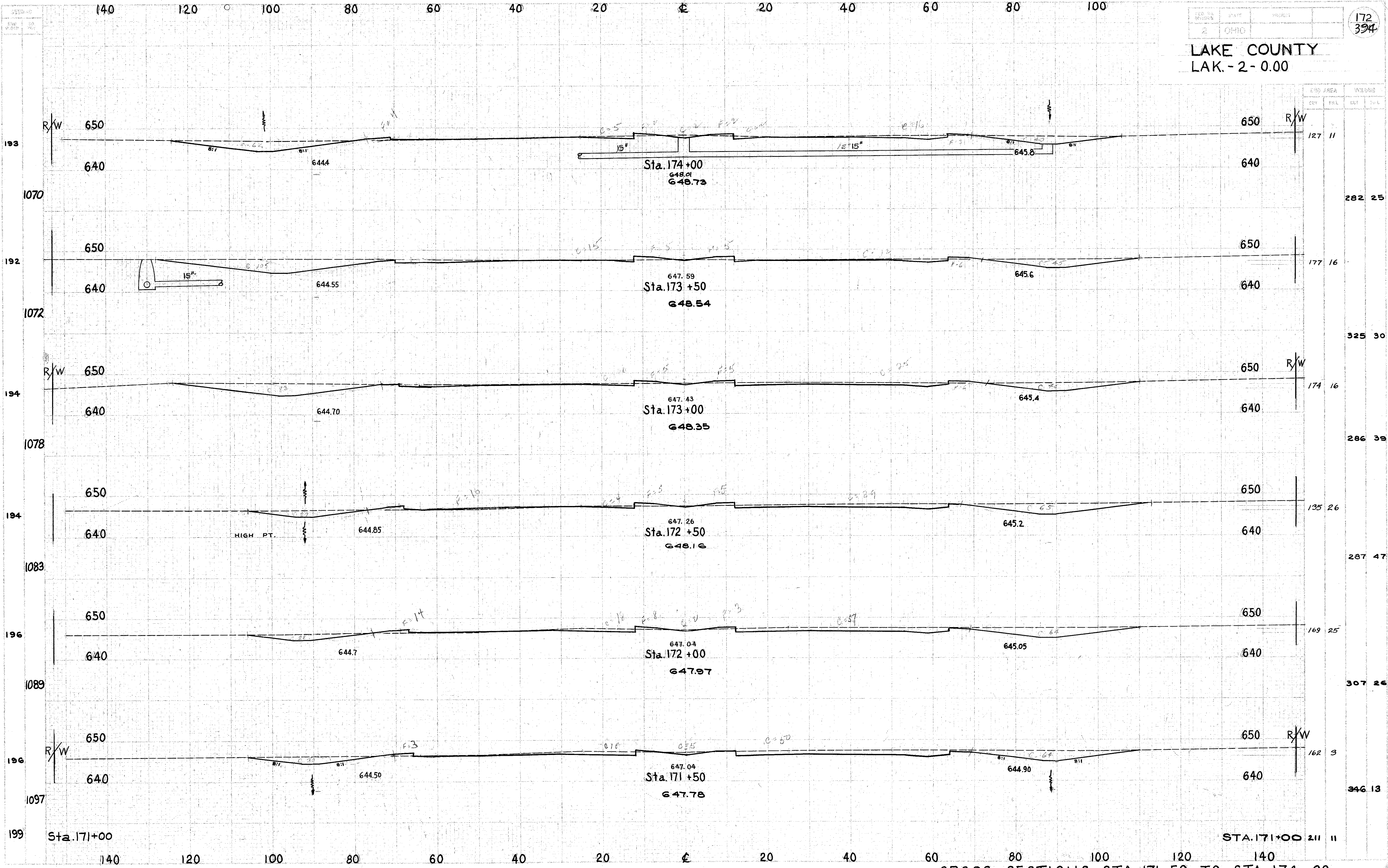
CROSS SECTIONS STA. 171+50 TO STA. 174+00
