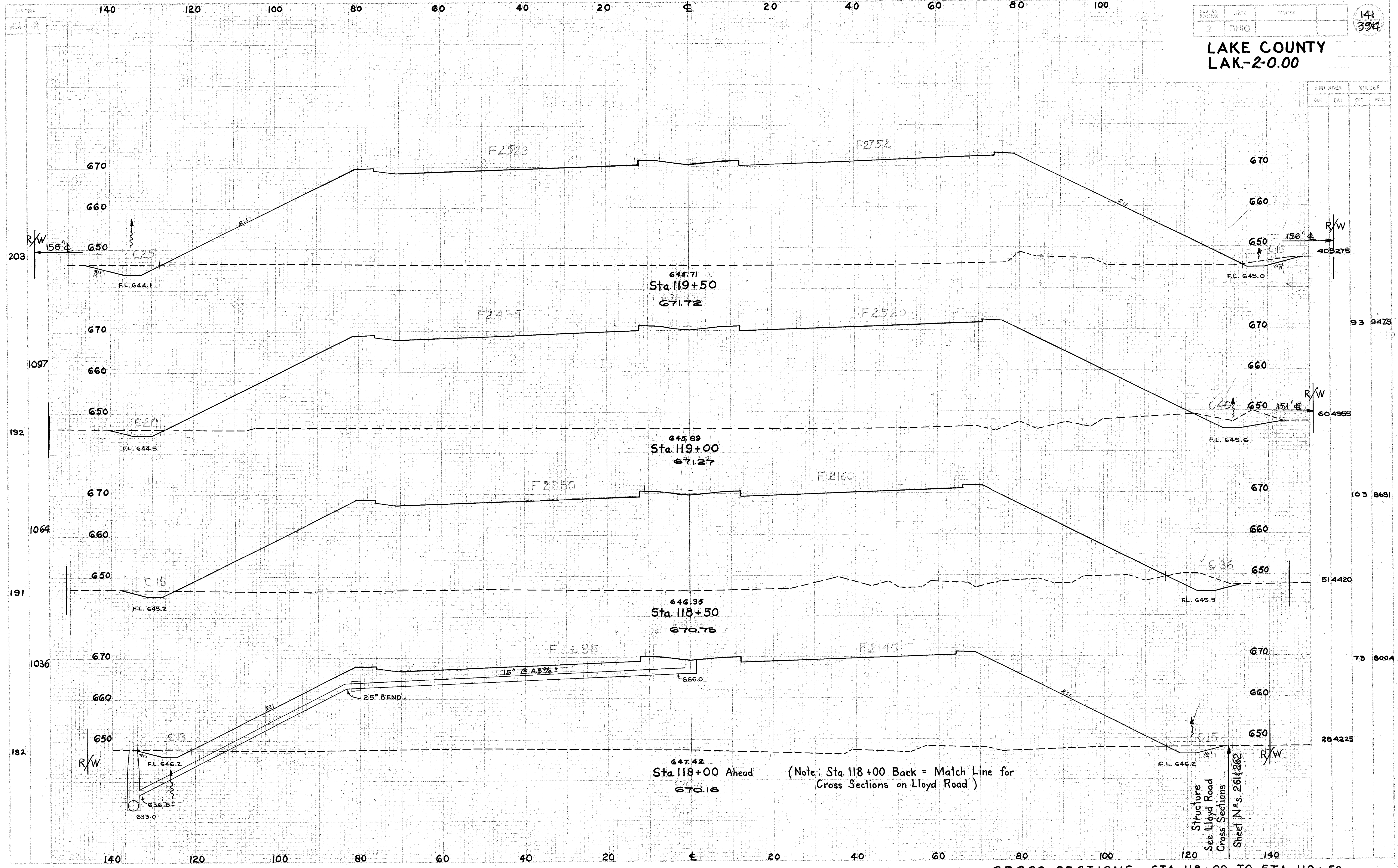
CROSS SECTIONS - STA. 118+00 TO STA. 119+50
