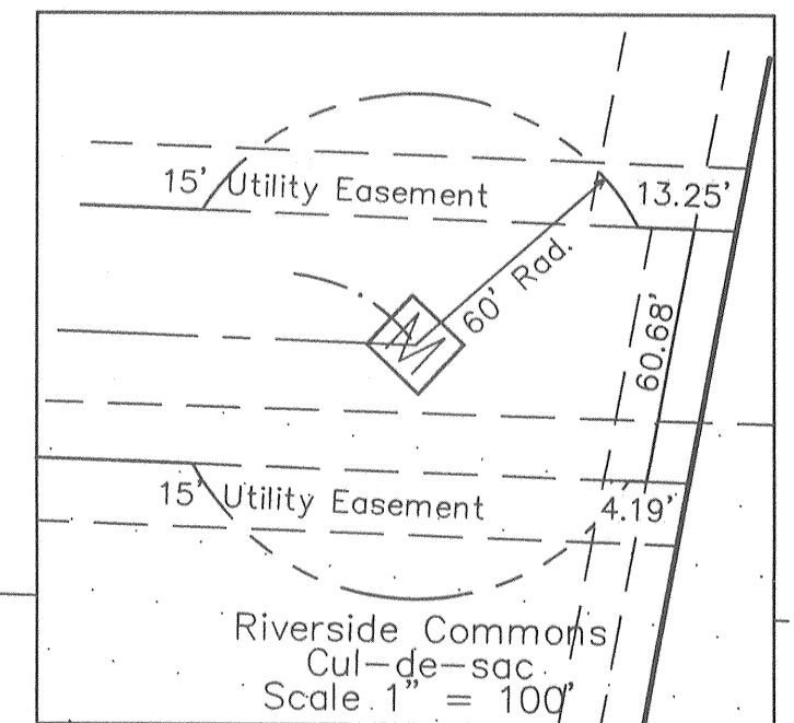
Riverside Commons Cul-de-sac Scale 1" = 100'
